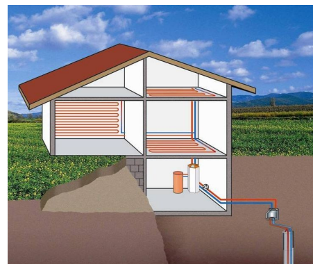
Bild: Mit einer Wärmepumpe wird über eine Tiefensonde dem Erdreich Erdwärme entnommen, mit der Wärmepumpe auf eine höhere Temperatur gebracht und über das Heizsystem in die Wohnräume geleitet.
